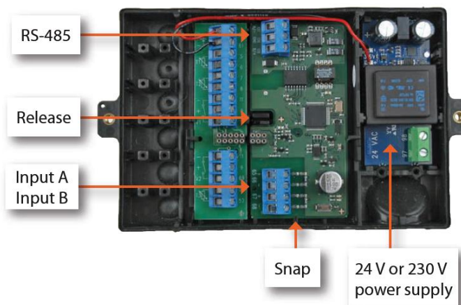
Modbus modul MULTICAL alaplapon
